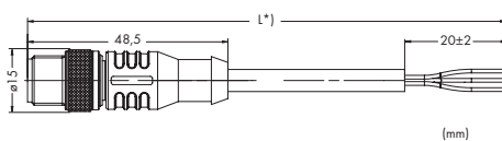
Штекер M12
