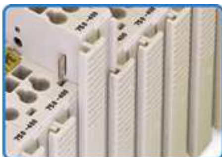
...надежное соединение "ласточкиным хвостом"
