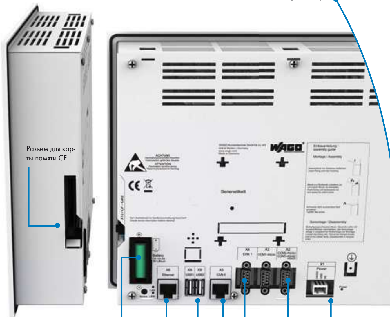
Батарея для буферизации данных в случае нарушения электропитания
