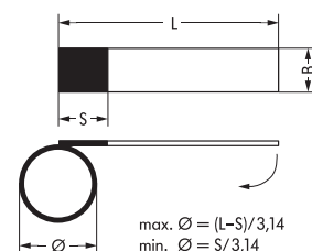
Размеры самоламинирующегося ярлыка
