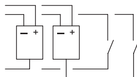
Дискретные входы X1 - X4 (два входа на соединитель) 1: 24 В 2: 24 В U_{IS} 3: 0 В U_{IS}
