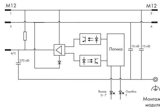
Дискретный выход X1 - X4
