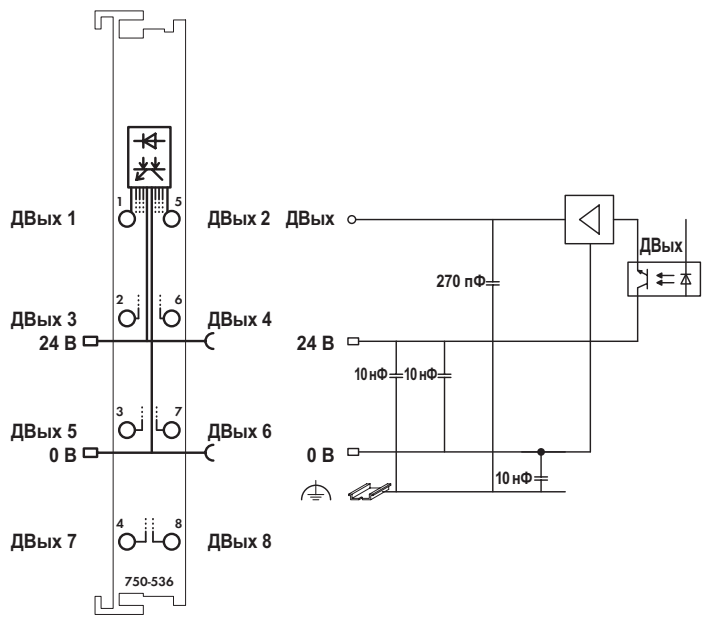
ПРИМЕЧАНИЕ: маркировка точек подключения (т.е. 1 - 8) не имеет отношения к распределению каналов
