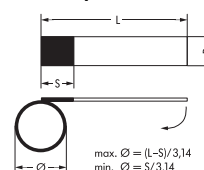
Размеры самоламинирующегося ярлыка
