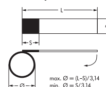
Размеры самоламинирующегося ярлыка
