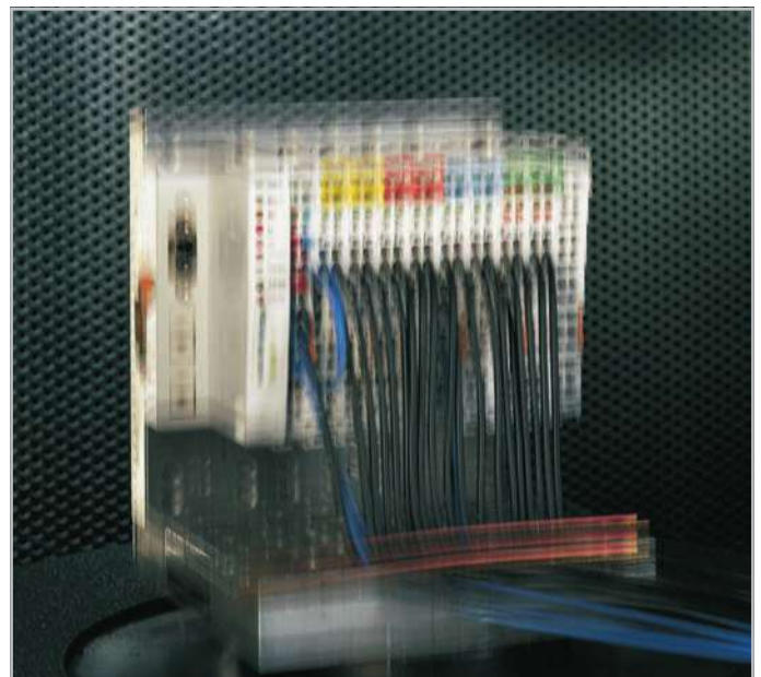
Испытания на вибрацию: WAGO-I/O-SYSTEM
