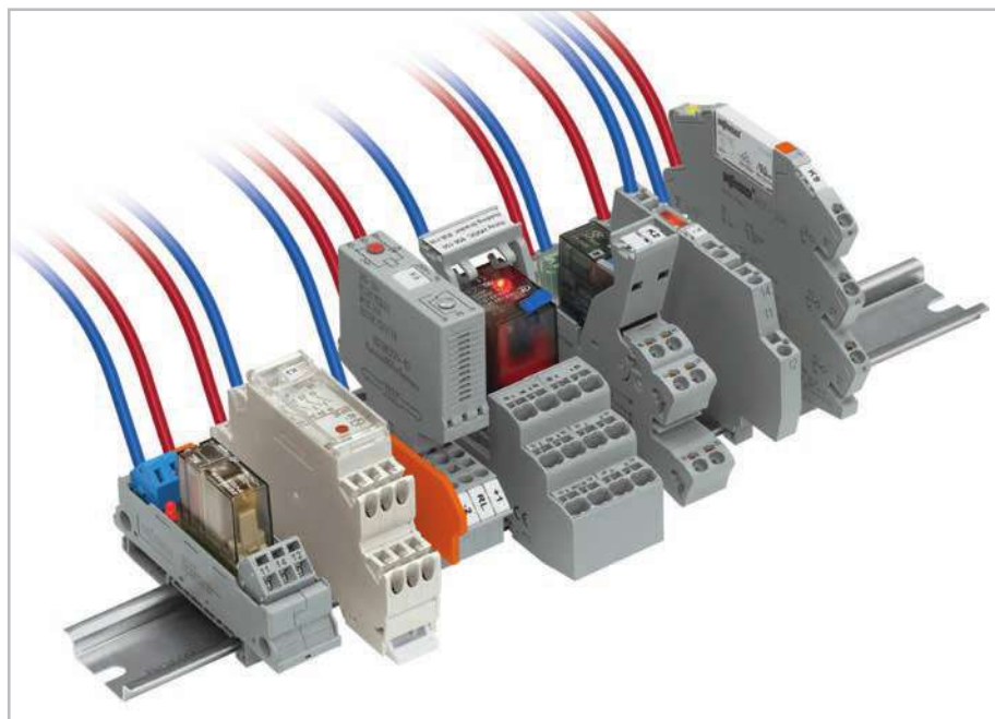
Подсоединение проводника методом фронтального монтажа
