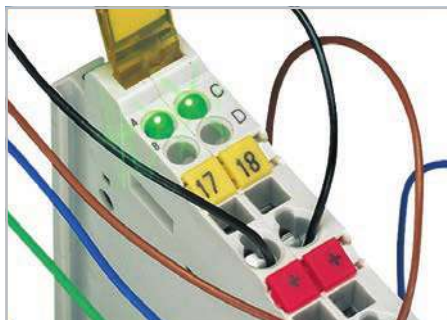
Диагностические и статусные светодиоды для безопасного ввода установки в эксплуатацию и контроля ее работы.
