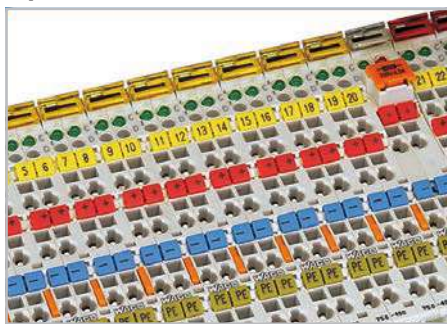
Маркировка зажимных устройств цветными мини-маркерами WSB
