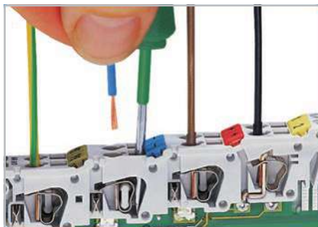
Виброустойчивые, быстрые и не требующие обслуживания соединения для проводников с сечением 0,08 ... 2,5 мм 2 (28 ... 14 AWG)
