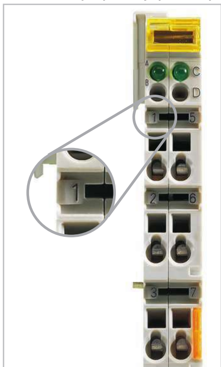
Точки соединения обозначаются с помощью выпоняемой на заводе печати.
