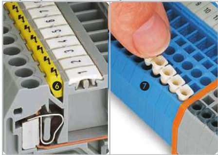
6 Защитная предупреждающая маркировка, устанавливаемая в слоты рабочего инструмента 7 Установка стопора для изоляции.
