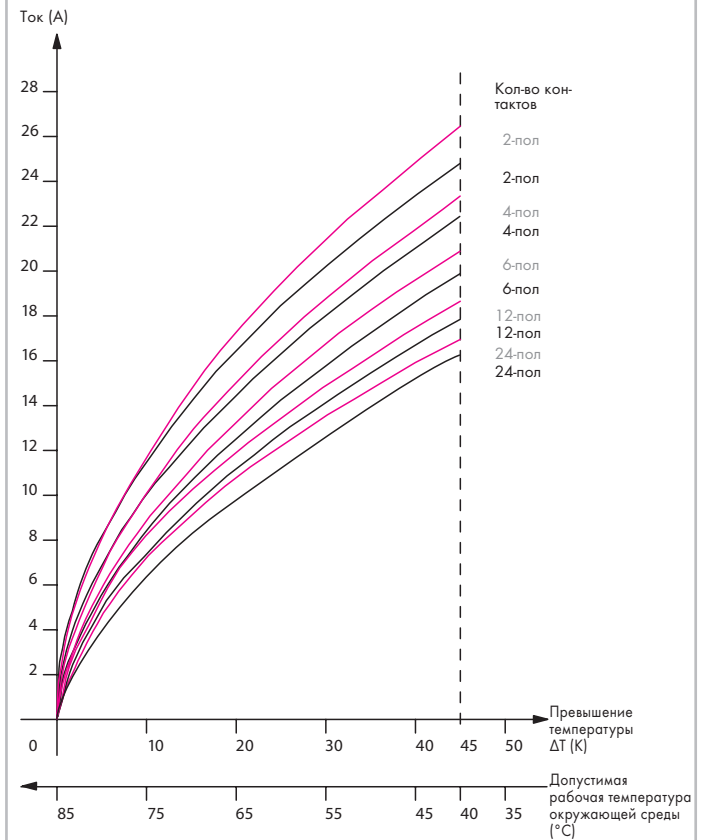
Вилки с прямыми выводами под пайку: 1 мм x 1 мм/1,2 мм x 1,2 мм MIDI Шаг контактов: 5 мм, 5,08 мм, 7,5 мм и 7,62 мм
