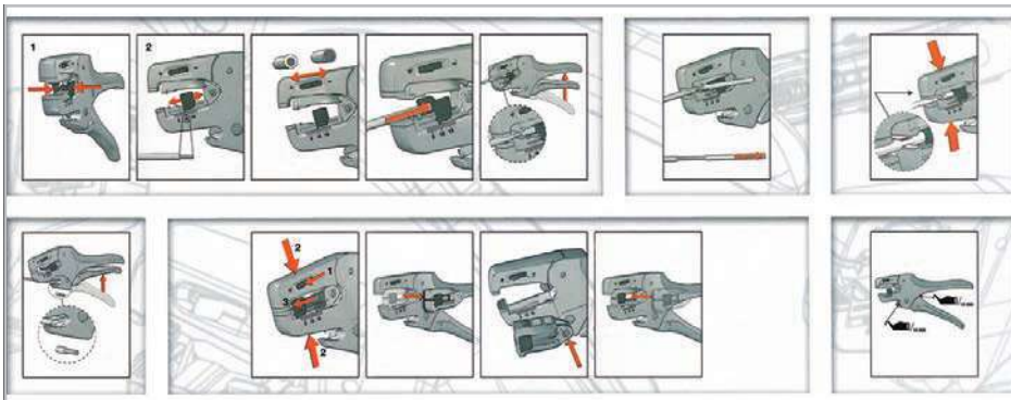
Обрезание проводника.
