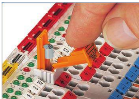
Функция в зафиксированном положении 2: простая замена предохранителя благодаря откидной крышке. Внимание: использовать только предохранители, на которые имеется допуск UL!
