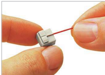
Зачистите одно-проводочные проводники на длину 5 ... 6 мм.
