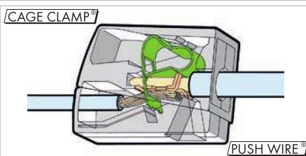
Страна монтажа: вставьте зачищенный одно-проводочный проводник в круглое отверстие до упора.
